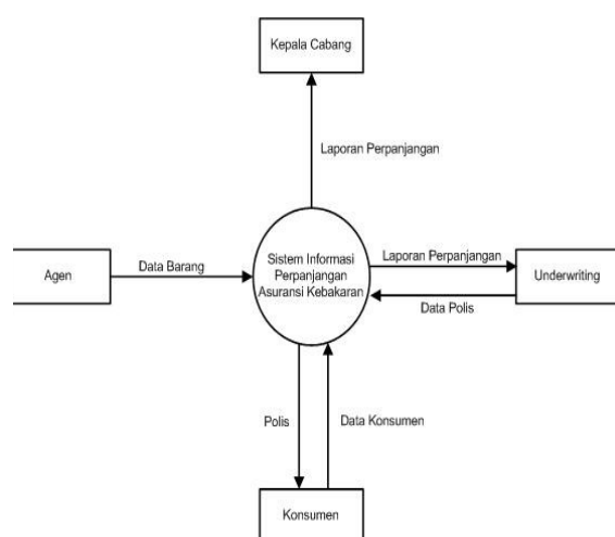
Gambar 3. Diagram Konteks
