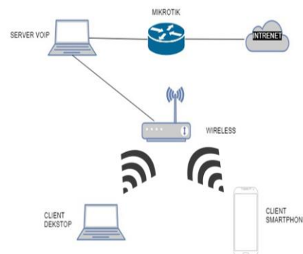
Gambar 2.2 Topologi Jaringan VoIP
